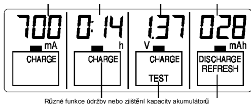
Různé funkce údržby nebo zjištění kapacity akumulátorů
